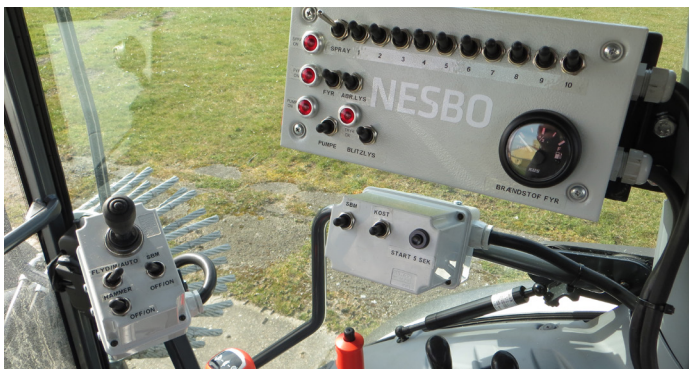
Overskuelig betjeningspanel monteret i kabine for effektiv drift
