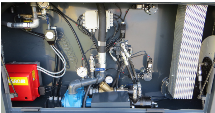
Enkelt og overskuelig opbygning af teknikrum for let betjening
