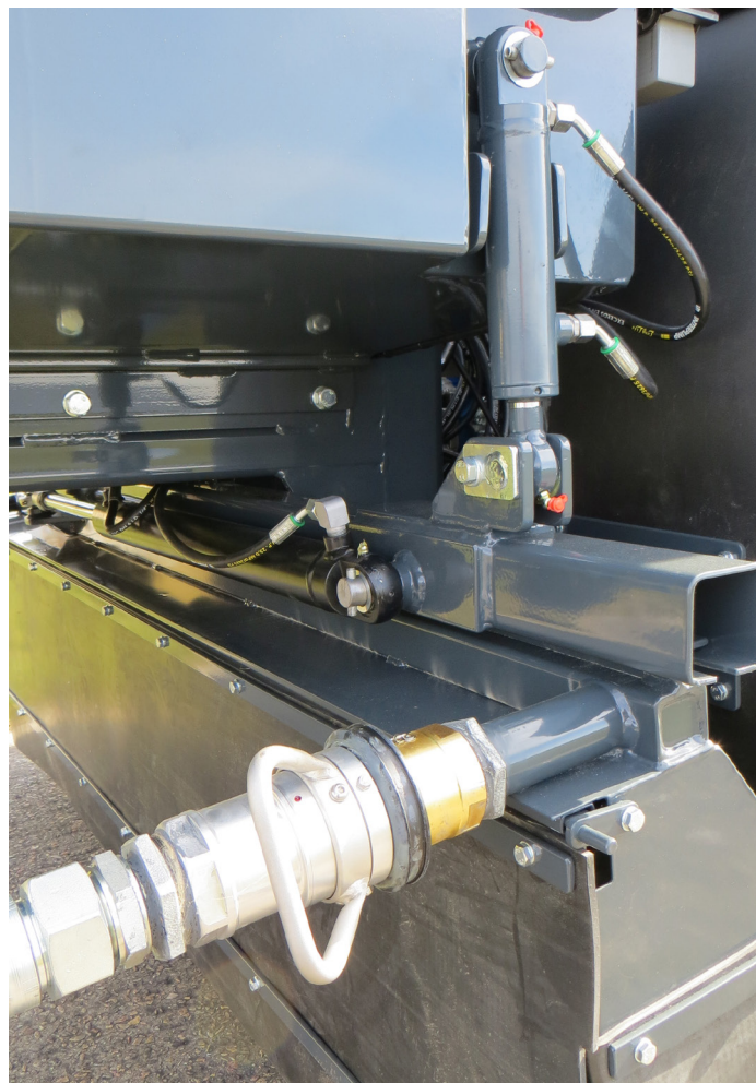
Fastmonteret tank med hydraulisk løft af bom, samt hydraulisk sideforskydning på i alt 600 mm højre/venstre
